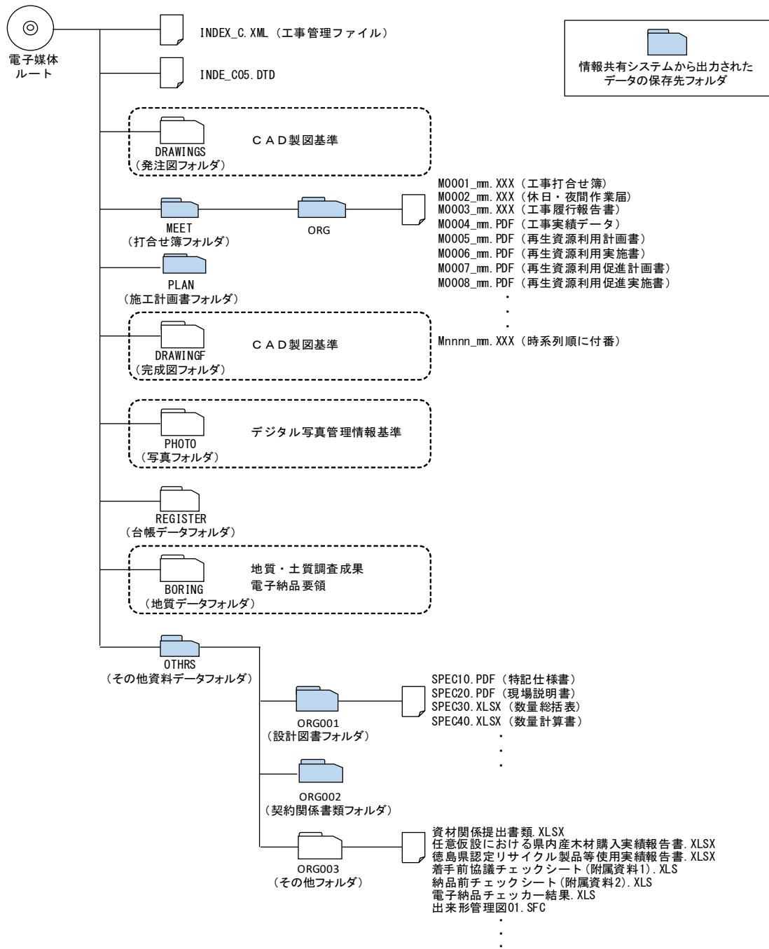
図1 フォルダ構成
